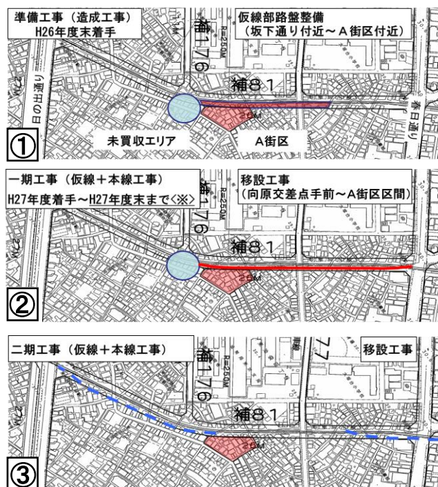
▲ 軌道工事の予定
