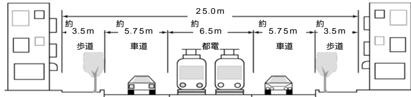
道路の構造 (標準断面)
